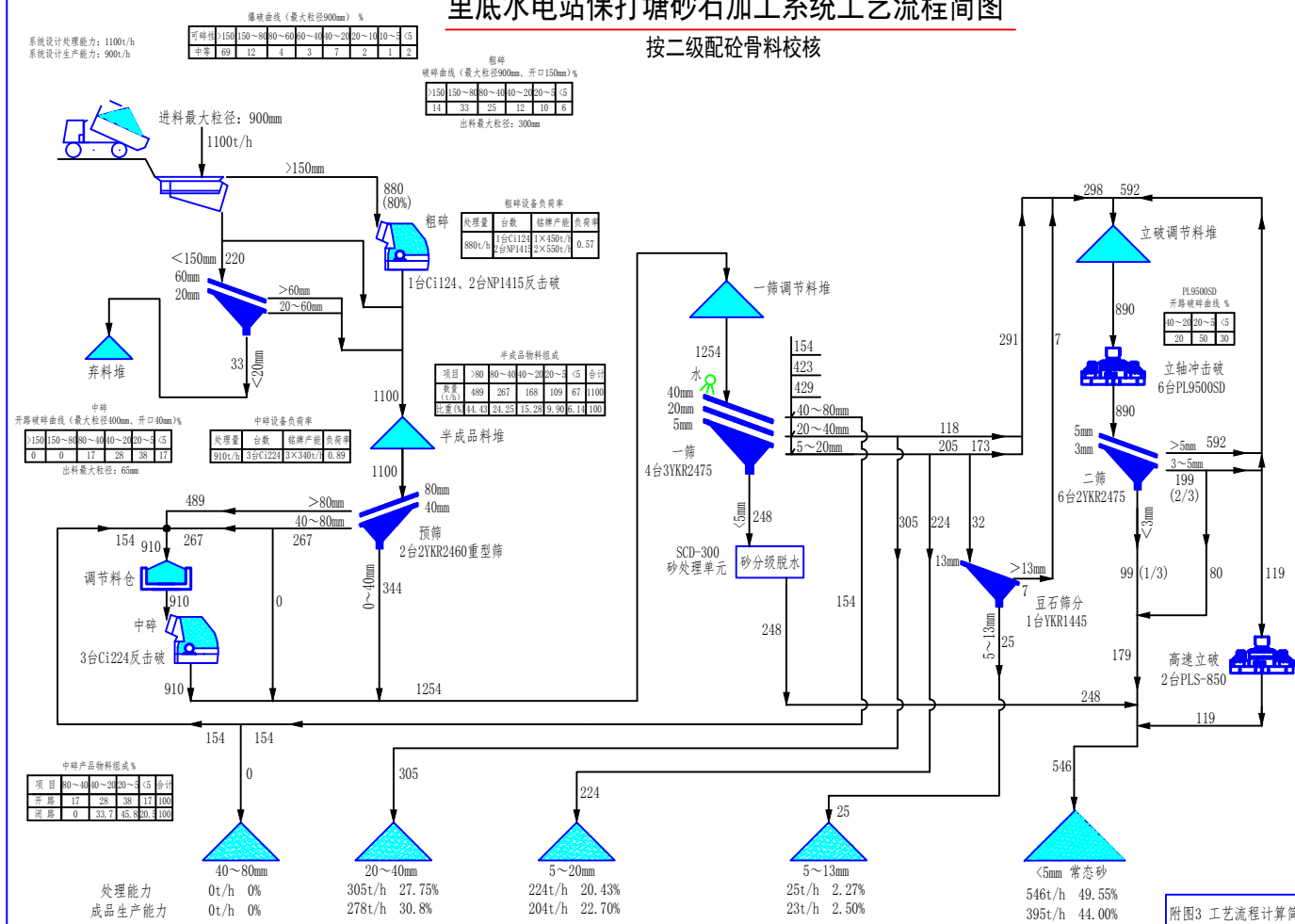
附图3 工艺流程计算简图2
